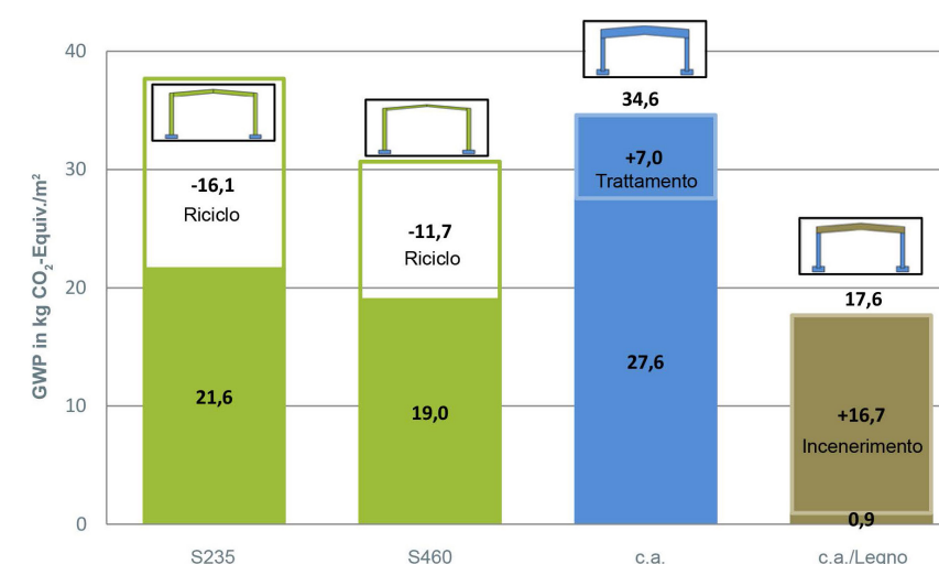
POTENZIALE DI RISCALDAMENTO GLOBALE PER LA FASE DI PRODOTTO SOMMATO AI COSTI E BENEFICI DA RICICLO (ACCIAIO), INCENERIMENTO (LEGNO) O TRATTAMENTO DELLE MACERIE (CALCESTRUZZO), PER UN EDIFICIO A TELAIO CON FONDAZIONI, MISURATO IN KG DI CO 2 EQUIVALENTI PER MQ DI SUPERFICIE CALPESTABILE. Fonte: Fondazione Promozione Acciaio - Analisi comparativa del ciclo di vita di un tipico edificio monopiano
